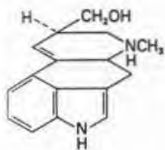
LYSERGOL
